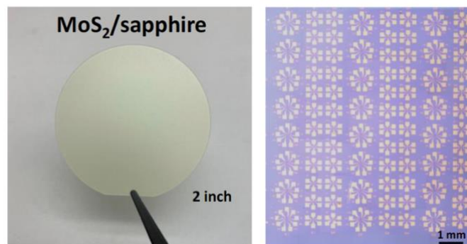
MoS 2 単結晶ウェハーとデバイス群
