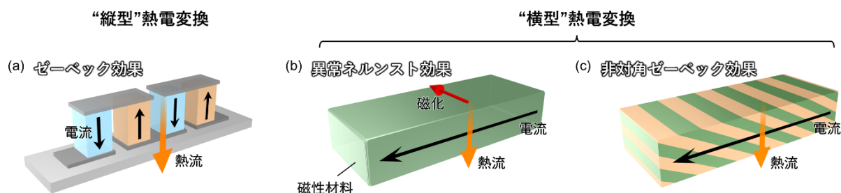
図1 (a) ゼーベック効果に基づく縦型熱電素子と、(b) 異常ネルンスト効果、(c) 非対角ゼーベック効果に基づく横型熱電素子の模式図
