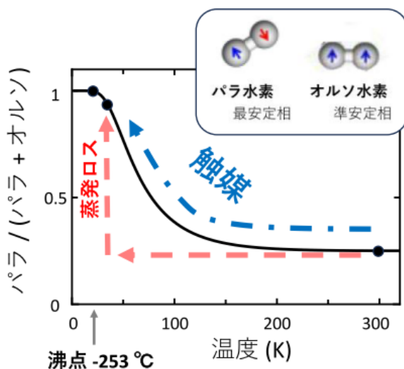
図1(上パネル)オルソ水素分子とパラ水素分子の模式図。水素原子の核スピンは、オルソ水素では平行に、パラ水素では反平行に配列している。(メインパネル)2つの水素分子の存在比の温度依存性の理想曲線。両者のエネルギー差は非常に小さいため、十分時間をかけて冷却すればオルソ水素はすべてパラ水素に変換されるが、急冷すると何割かのオルソ水素がパラ水素に変換されないまま液化水素中に残り、その結果、赤破線のように蒸発ロスが生じる。そのため、変換を迅速化する触媒の開発が課題となっている。
