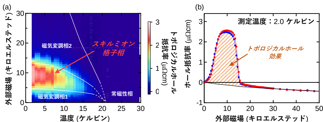
図2 磁気スキルミオン格子状態でのトポロジカルホール効果
