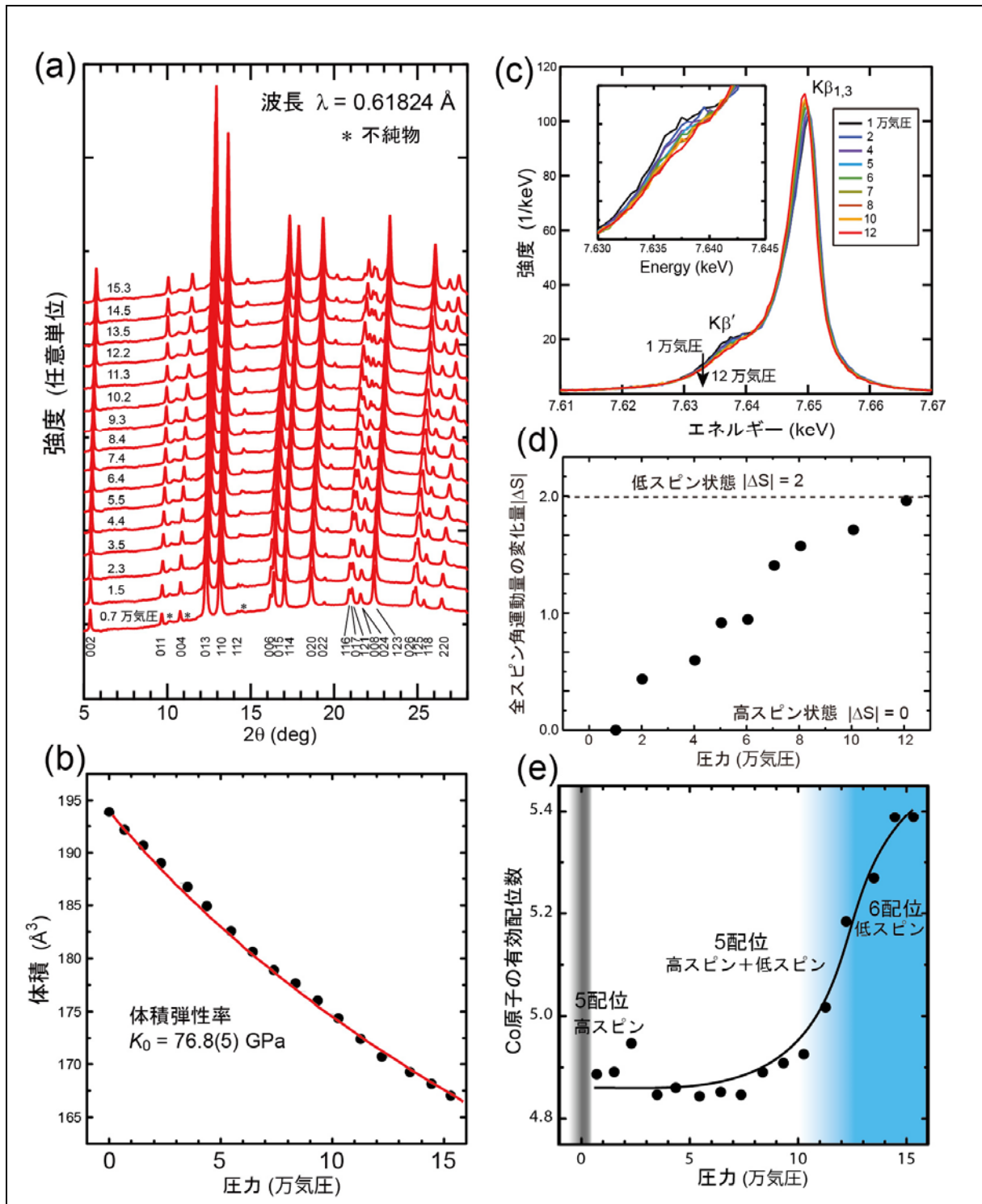
図2. (a) \text{Sr}_2\text{CoO}_3\text{F} の高压放射光粉末 X 線回折パターンの圧依存性。測定圧力内では結晶対称性 ( I4/mmm ) は維持されている。(b) 体積の圧力変化。(c) \text{Sr}_2\text{CoO}_3\text{F} の Co K\beta X 線発光スペクトルの圧力依存性。挿入図はサテライトピーク ( K\beta' ) の拡大図。スピン状態が小さいほど、サテライトピーク強度は弱く、メインピーク ( K\beta_{1,3} ) の位置が低エネルギー側にシフトする。(d) スペクトルデータから見積もられた Co の全スピン角運動量の変化。12 万気圧で低スピン状態に完全に転移する。(e) 各圧力における \text{Sr}_2\text{CoO}_3\text{F} の Co サイトの有効配位数。10 万気圧以上で配位数が急増加し、14.5 万気圧で飽和する傾向を示す。14.5 万気圧における有効配位数の値は 5.4 であり、 \text{LaMnO}_3 の軸方向に歪んだ \text{MnO}_6 八面体の有効配位数 5.23 よりも大きいことから、Co サイトは実質 6 配位状態と見なすことができる。
