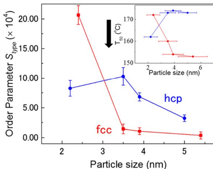
図 1. 面心立方格子構造(fcc)タイプの Ru ナノ粒子と六方最密充填構造(hcp)タイプの Ru ナノ粒子の原子スケールの逆モンテカルロ(RMC)モデリングの結果から得られた構造秩序パラメーター (Order Parameter) のナノ粒子のサイズとの関係。各 Ru ナノ粒子のサイズは透過型電子顕微鏡像の結果から求めました。挿入図は粒子サイズによる CO 触媒活性の変化を示している。(図中右上) 触媒活性の尺度である T_{50} は CO の反応率が 50% に達する温度を示しますので、 T_{50} が低い(矢印の下側方向)ほど高い触媒活性を持っていることを示します。
