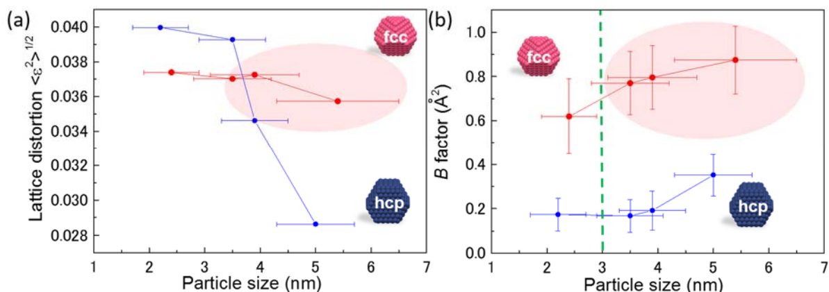
図 3. fcc タイプの Ru ナノ粒子と hcp タイプの Ru ナノ粒子の平均構造(長周期構造)を解析した結果。(a)粒子サイズ(Particle size)による Ru ナノ粒子の原子がもっとも密にある原子面の格子歪(Lattice distortion)の変化。(b)粒子サイズによる Ru ナノ粒子の温度因子(B factor)の変化。(a)と(b)の赤色の楕円は相対的に高い触媒活性を発揮する Ru ナノ粒子を示しています。
