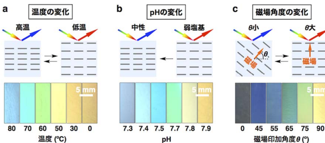
図5 環境の変化に応じて構造色を変化させる動的フォトニック構造体
