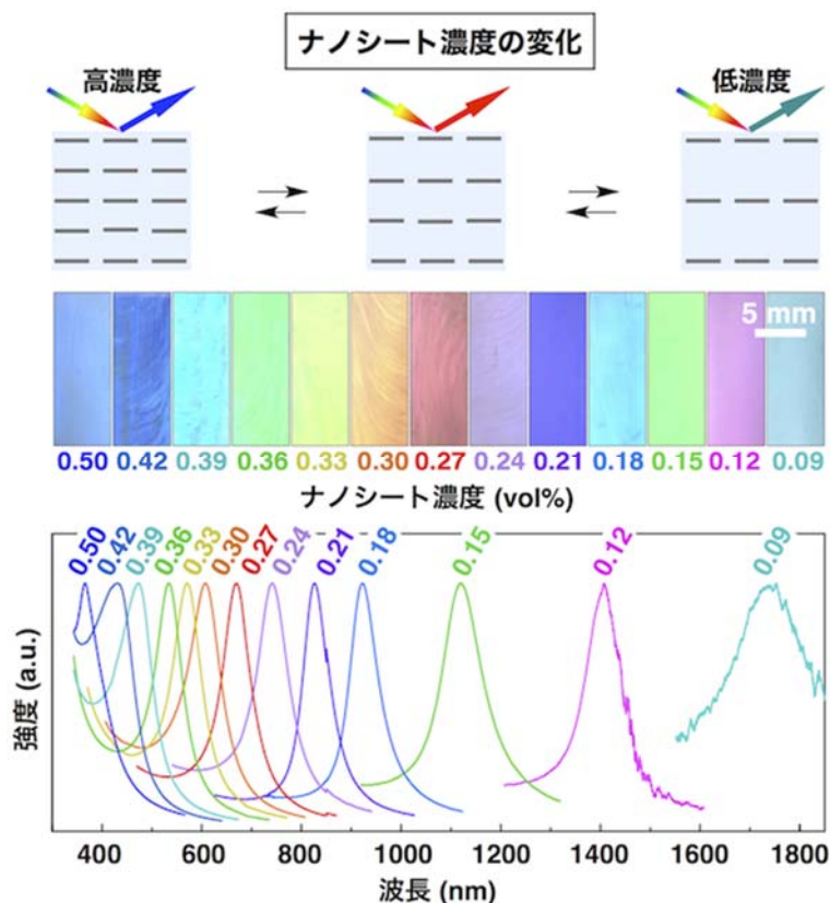
図 3 紫外光領域から近赤外光領域にわたり反射波長を制御可能な動的フォトニック構造体濃度を調節することにより、酸化チタンナノシートの水分散液の反射波長は、全可視光領域のみならず紫外光領域（370nm）から近赤外光領域（1,750nm）にわたる広い範囲で連続的に制御できる。分散液の外観（中段）ならびに反射スペクトル（下段）。
