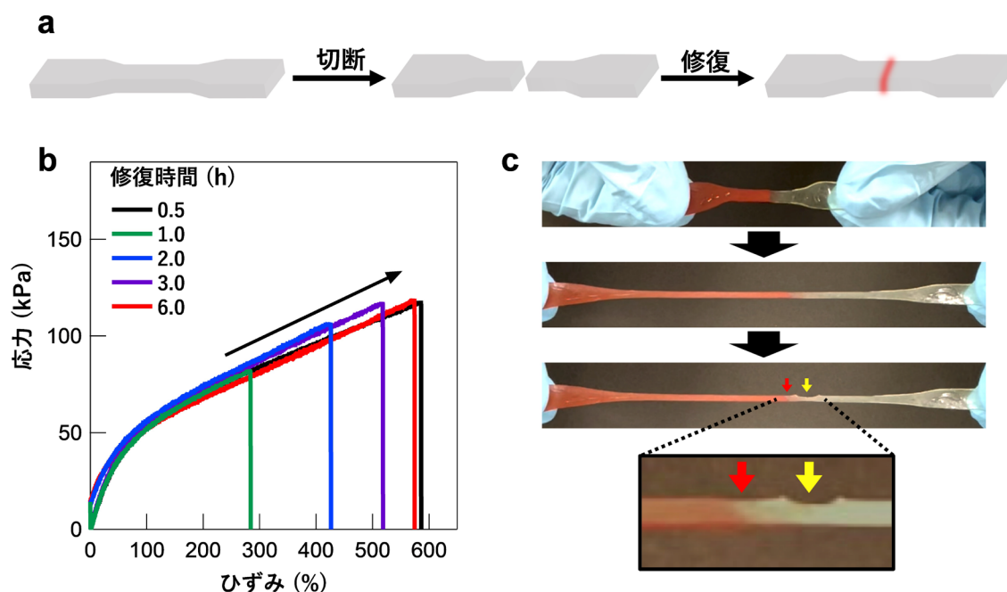
図3. (a)自己修復試験の模式図。(b)修復時間の異なる超高分子量ゲルの応力-ひずみ曲線。(c)修復6時間後の超高分子量ゲルの伸長写真。視認性を良くするために、着色を加えた試験片と着色していない試験片を切断し、片方ずつの切断面を接着させている。写真から接着面(赤矢印)ではない点で破断が始まっております(黄色矢印)、切断面の自己修復が十分進んでいることが分かる。
