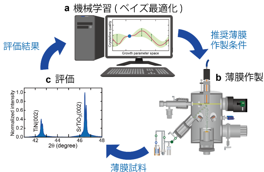
図 機械学習を導入した Closed-loop operation による薄膜作製パラメーター最適化の概略
