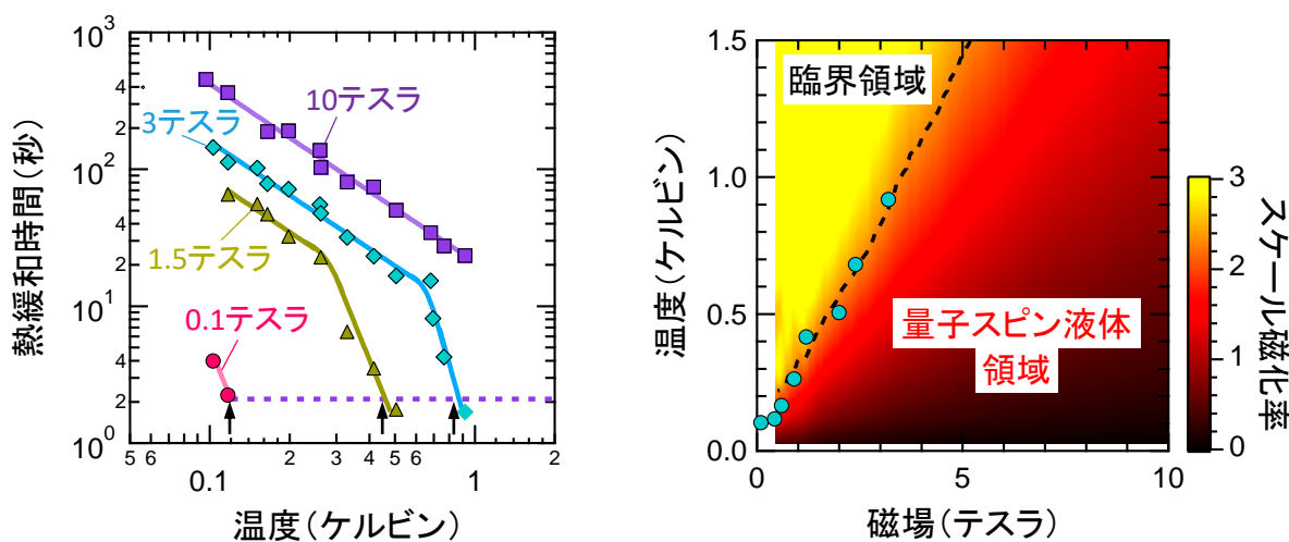
図2. (左) 電子スピン系から格子系への熱緩和時間の温度依存性。極低温・磁場中において、温度減少に伴って熱緩和時間が急激に長くなることが分かります。(右) 温度—磁場相図。共同研究グループが、以前、磁化率測定によって決定した相図中の赤色の領域（量子スピン液体領域）で、熱緩和時間が急激に長くなることがわかりました。このメカニズムは現在不明であり、研究が進行中です。
