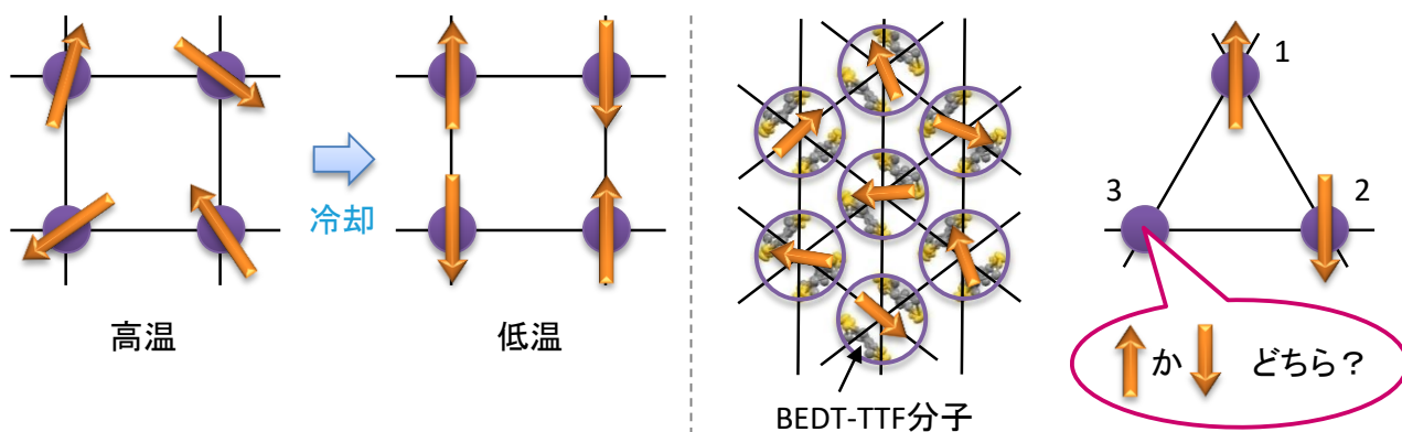
図1. (左) 磁性体内部での電子スピンの様子。紫色の丸が原子を、橙色の矢印がその原子の電子のスピンを示しています。原子上にいる電子のスピンは、高温では熱的に揺らいでおり、バラバラな方向を向いています（スピン液体状態）。磁性体を冷却して熱揺らぎを小さくすると、スピンは向きを揃えて整列して秩序を作ります（スピン固体状態）。この図では、隣り合うスピン同士を反対向きに揃えようとする相互作用（反強磁性的相互作用）を想定しています。
