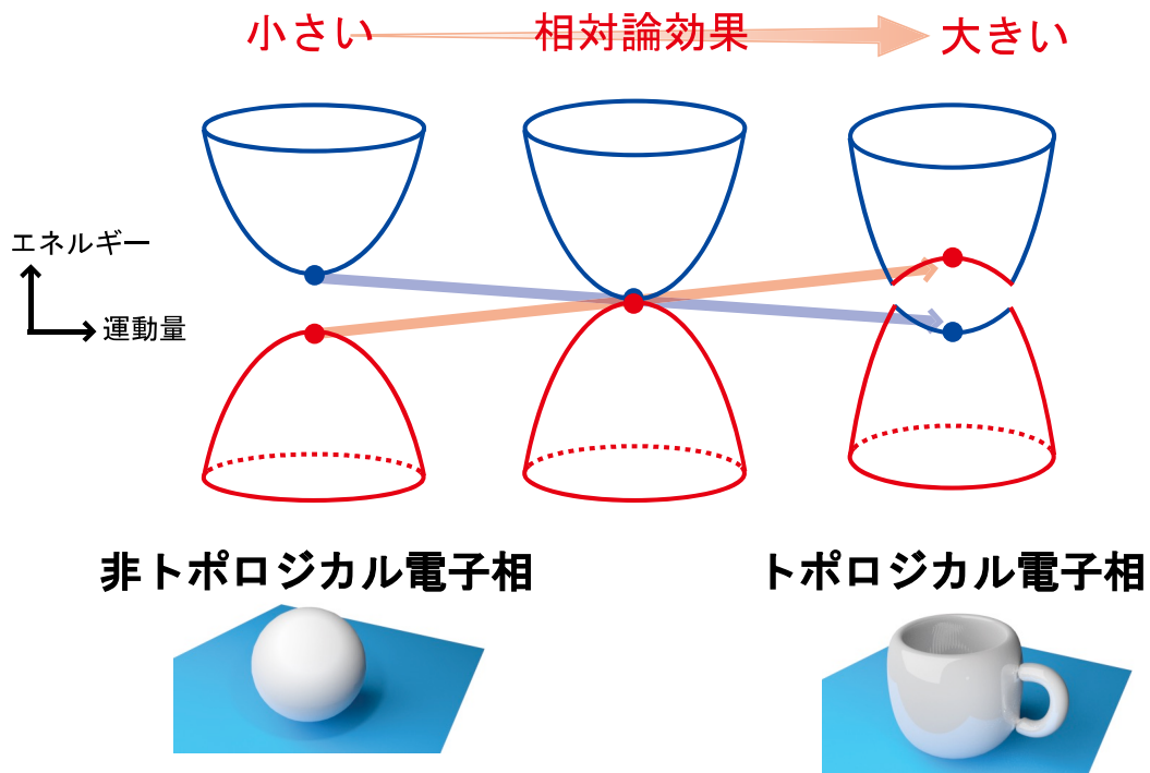
図1 : 本研究で観測された相対論効果によるトポロジカル相転移。
