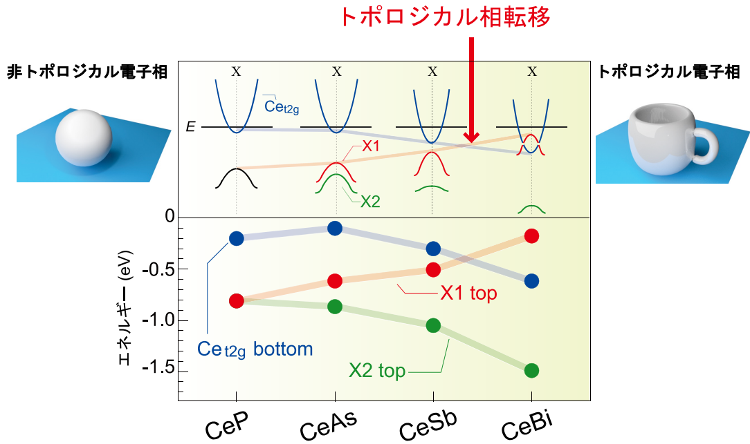
図2：軟 X 線を用いた光電子分光で観測されたセリウムモノプニクタイトの物質群の電子構造とトポロジカル相転移。プニクトゲン元素がリン (P) からビスマス (Bi) になるにつれて相対論効果が大きくなる。CeP から CeBi まで系統的に電子構造を観測する事で、その相対論効果による電子構造の変化に注目した。その結果、CeSb から CeBi になるとバンドの反転がおりトポロジカル相転移が発生していることがわかった。この物質群で最も相対論効果の大きい CeBi がトポロジカル電子相であることがわかった。
