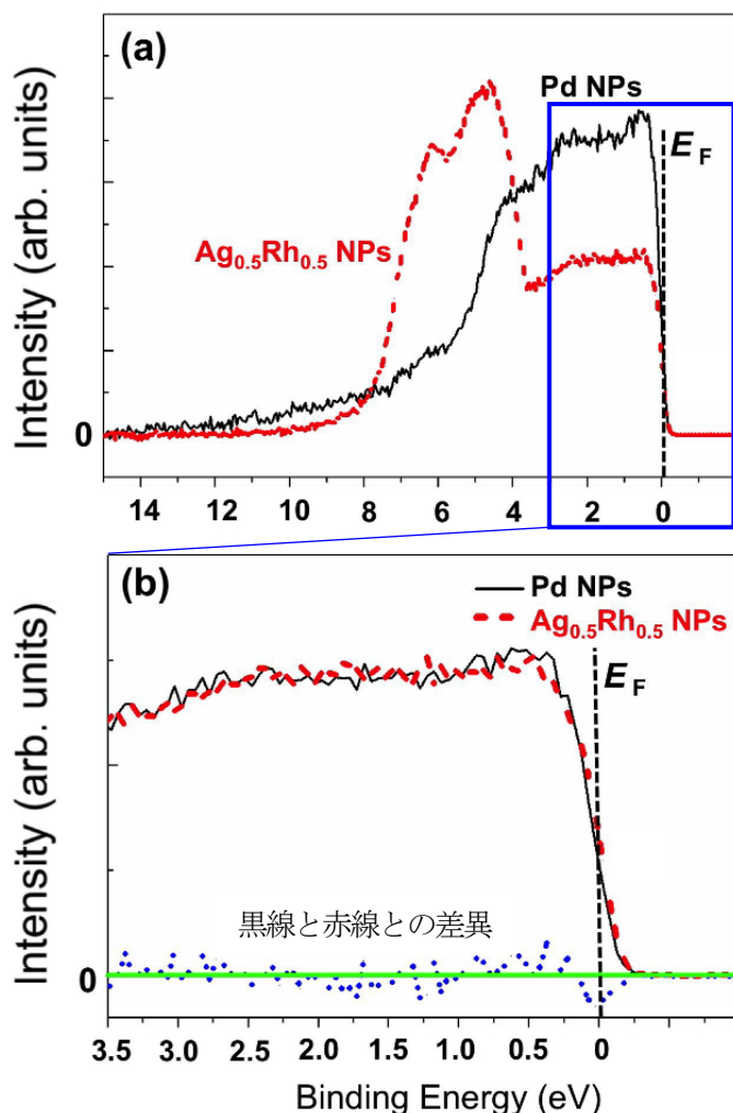
図 Pdナノ粒子と \text{Ag}_{0.5}\text{Rh}_{0.5} 合金ナノ粒子の高輝度放射光光電子分光スペクトルの比較。(a) 0-15eVの結合エネルギーの範囲における \text{Ag}_{0.5}\text{Rh}_{0.5} 合金ナノ粒子(赤破線)とPdナノ粒子(黒実線)の高輝度放射光分光による価電子帯スペクトル。 \text{Ag}_{0.5}\text{Rh}_{0.5} 合金の強度はPdの約半分。(b)0-3.5eVの結合エネルギーの範囲を拡大した \text{Ag}_{0.5}\text{Rh}_{0.5} 合金ナノ粒子(赤破線:強度をPdに合わせた拡大)とPdナノ粒子(黒実線)の価電子帯スペクトル。青い点線は、 \text{Ag}_{0.5}\text{Rh}_{0.5} 合金ナノ粒子の拡大されたスペクトル、Pdナノ粒子のスペクトルとの差異を示しています。 E_F はフェルミエネルギー。
