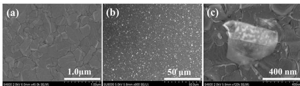
図2 金基板に担持したBNナノシートの電子顕微鏡写真
