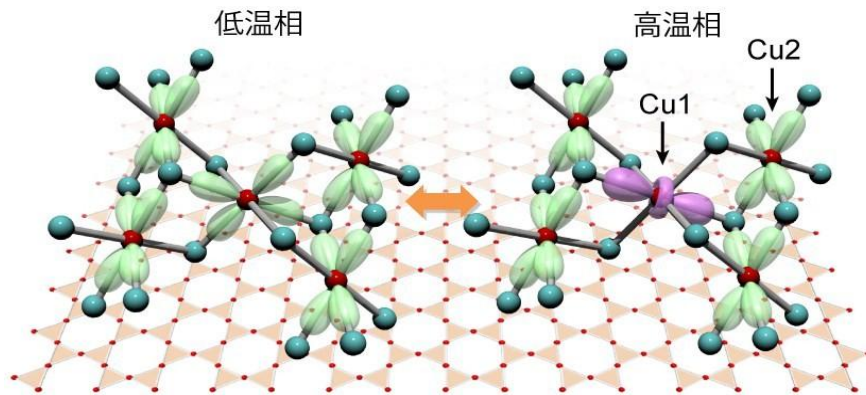
図2 銅鉍物ボルボサイト ( \text{Cu}_3\text{V}_2\text{O}_7(\text{OH})_2 \cdot 2\text{H}_2\text{O} ) の軌道スイッチング カゴメ格子上のCu1サイトにおいて、不対電子が入る d 軌道は、相転移温度 T_S = 310 \text{ K} を境界にして、 x^2-y^2 (低温相：左) から 3z^2-r^2 (高温相：右) へと切り替わります。これは、一種の秩序・秩序転移であり、「軌道スイッチング」と名付けられました。
