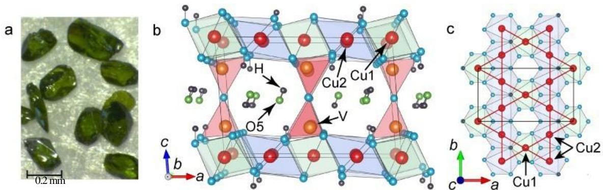
図1 銅鉍物ボルボサイト ( \text{Cu}_3\text{V}_2\text{O}_7(\text{OH})_2 \cdot 2\text{H}_2\text{O} ) の結晶構造 (a) 単結晶の実体顕微鏡写真、(b) b 軸方向から見た全体像、(c) c 軸方向から見たカゴメ格子層。
