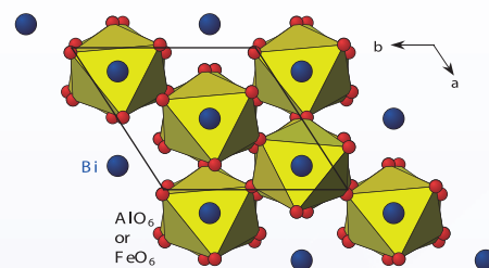
強誘電体 BiAlO 3 又は マルチフェイロック BiFeO 3 の結晶構造
