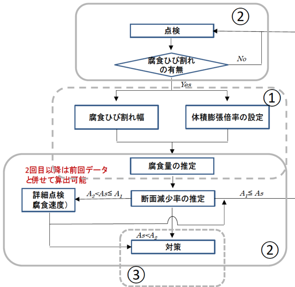
図1 腐食ひび割れと構造耐荷力に着目した管理フロー(京都大学 宮川豊章)と各サブクラスターの研究項目
