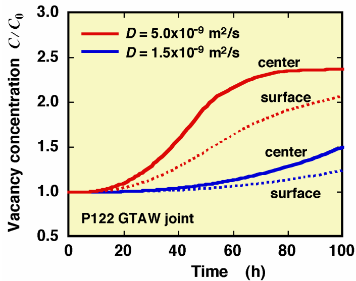
多軸応力下での原子空孔拡散・凝集の計算例
