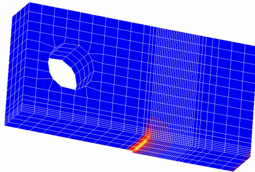
解析対象のCT試験片
