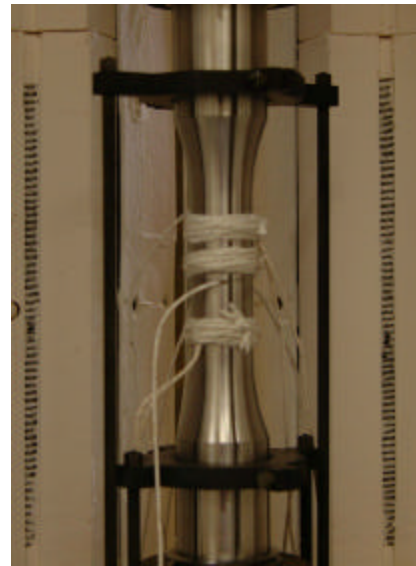
大型CT試験片によるき裂成長試験 大型環状切欠試験片のき裂成長試験
