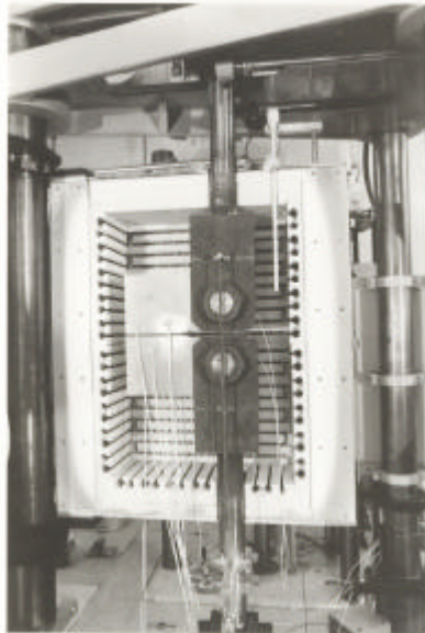
大型CT試験片によるき裂成長試験 大型環状切欠試験片のき裂成長試験
