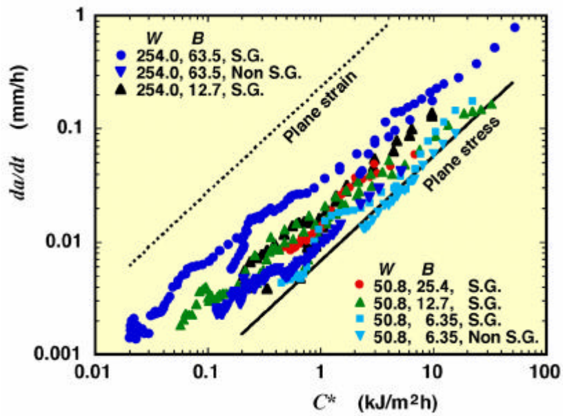
き裂成長速度に及ぼす試験片板厚の効果
