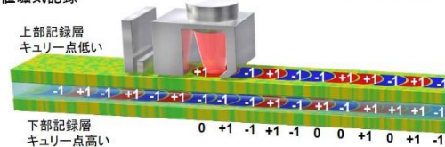
多値磁気記録
