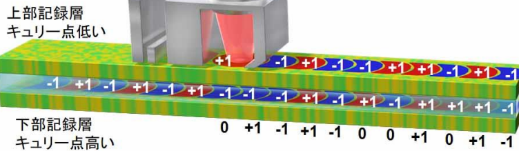
図1(a)現行のHAMR方式及び(b)3次元の磁気記録方式の模式図。3次元磁気記録方式では各記録層のキュリー一点に100K程度の差を付け、書き込み時のレーザー出力を調節することで各層の書き込みを行います。
